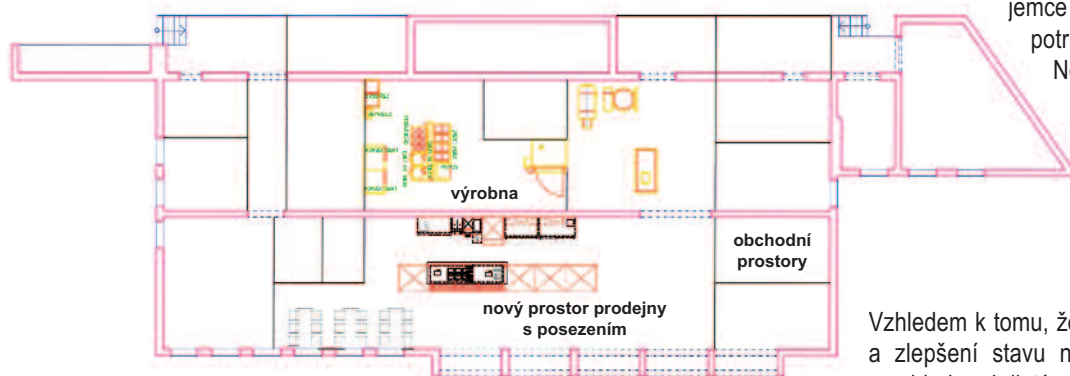
Návrh nové dispozice rekonstruované budovy potravin
