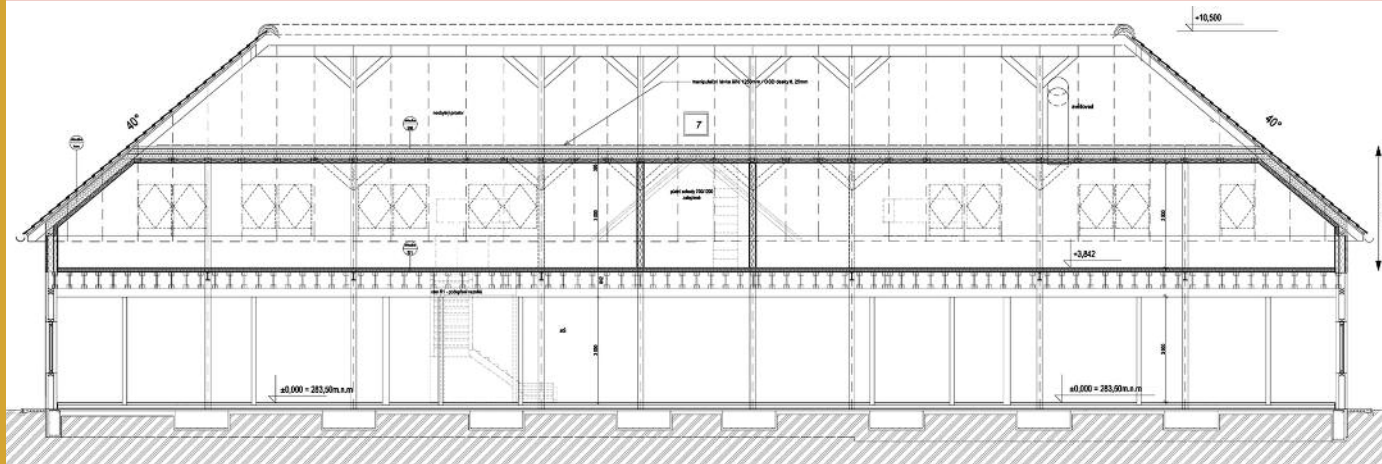
PODÉLNÝ ŘEZ
