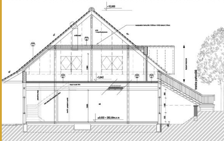
PŘÍČNÝ ŘEZ
